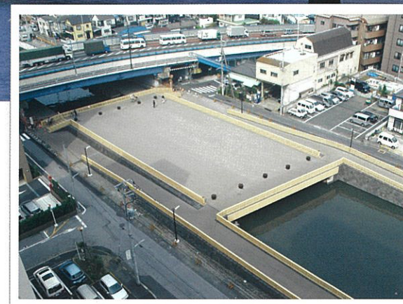
江戸川区新川広場橋(環七)仮設工事(その1) 東京都江戸川区 施工期間:平成22年4月~5月
